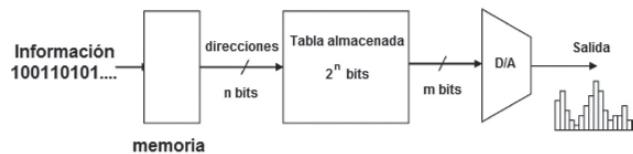
Figura 5. Diagrama esquemático del pre-compensador electrónico usado en nuestras investigaciones.
