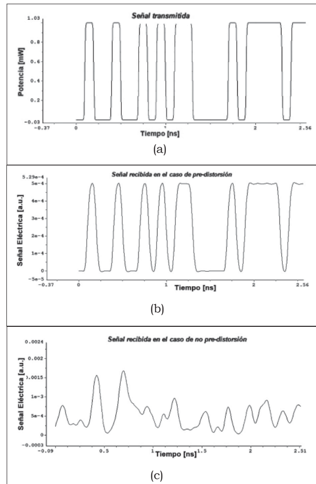
Figura 9. Comparación de las señales en el transmisor (a), recepción con pre-distorsión en la transmisión (b) y la recepción sin pre-distorsión en la transmisión (c).
