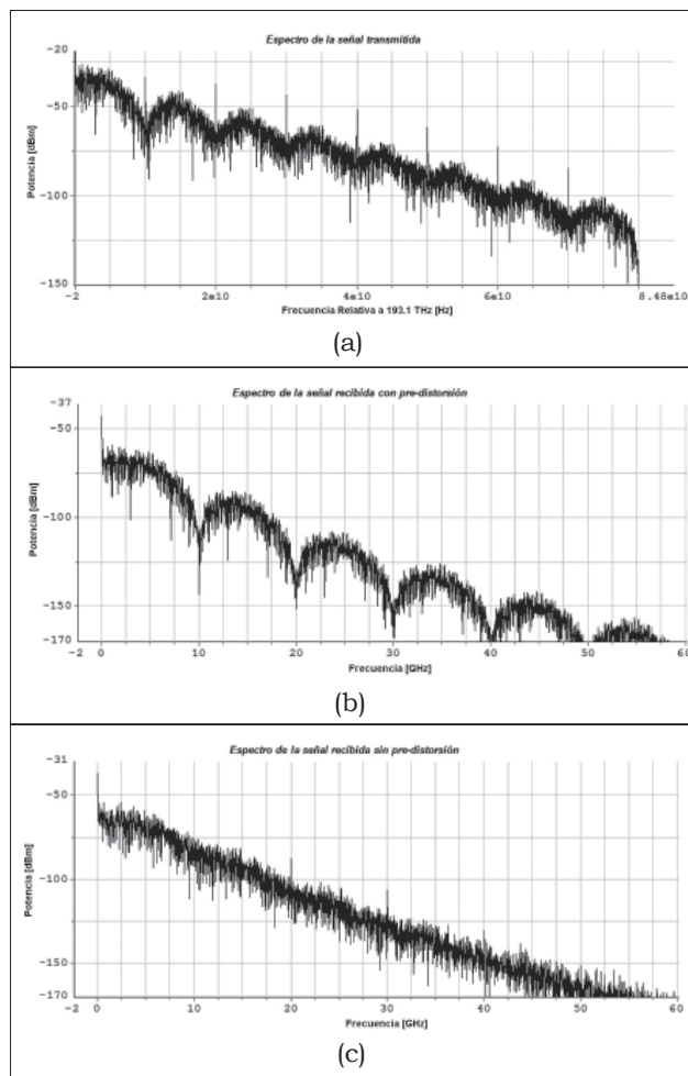
Figura 11. Espectros de la señal transmitida (a), señal recibida con pre-distorsión electrónica (b) y señal recibida sin pre-distorsión electrónica (c).
