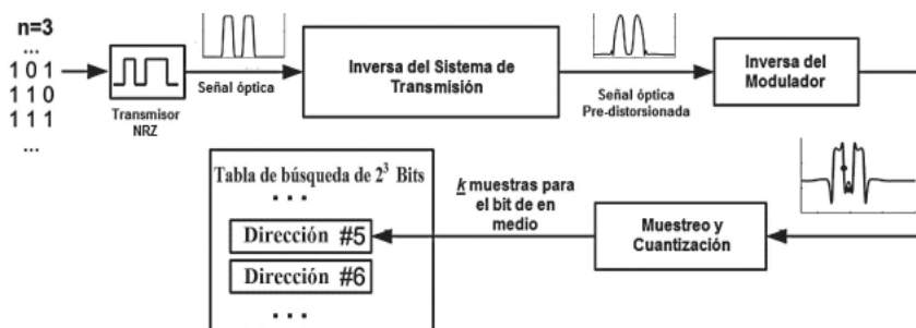
Figura 7. Ejemplo del cálculo de la tabla de búsqueda de dimensión 2^3 .
