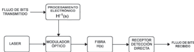
Figura 3. Diagrama a bloques de un enlace por fibra óptica con pre-compensación en el transmisor de la señal.
