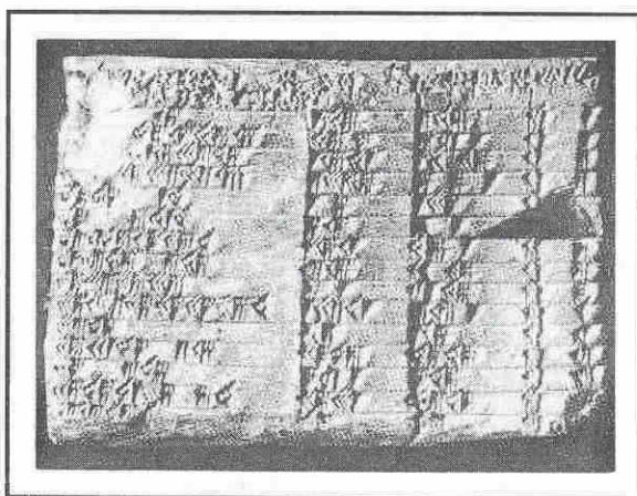
Tablilla babilónica
