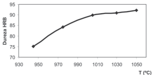
Figura 8. Dureza de la pasta seleccionada respecto a la temperatura de cocción.
