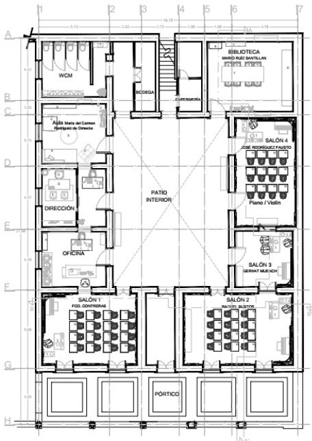
IMAGEN 1: Planta arquitectónica de la Escuela de Música
