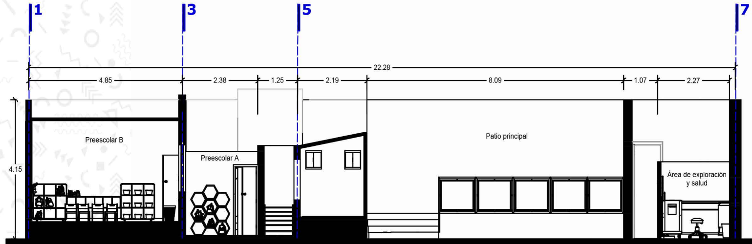
Corte E - E'
