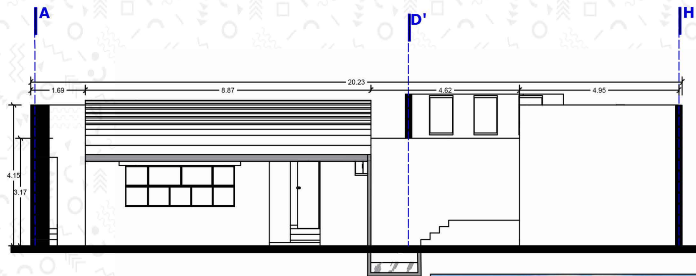
Corte Fachada
