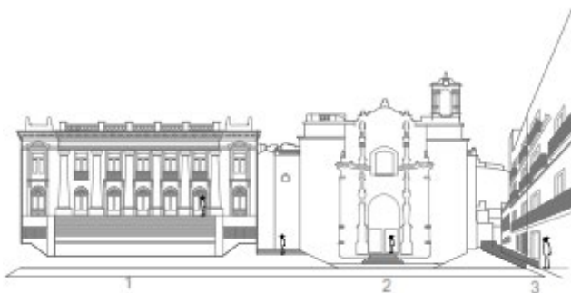
IMAGEN 2 Fachada suroeste: Teatro Juárez y Templo de San Diego, dibujo en auto-CAD.
