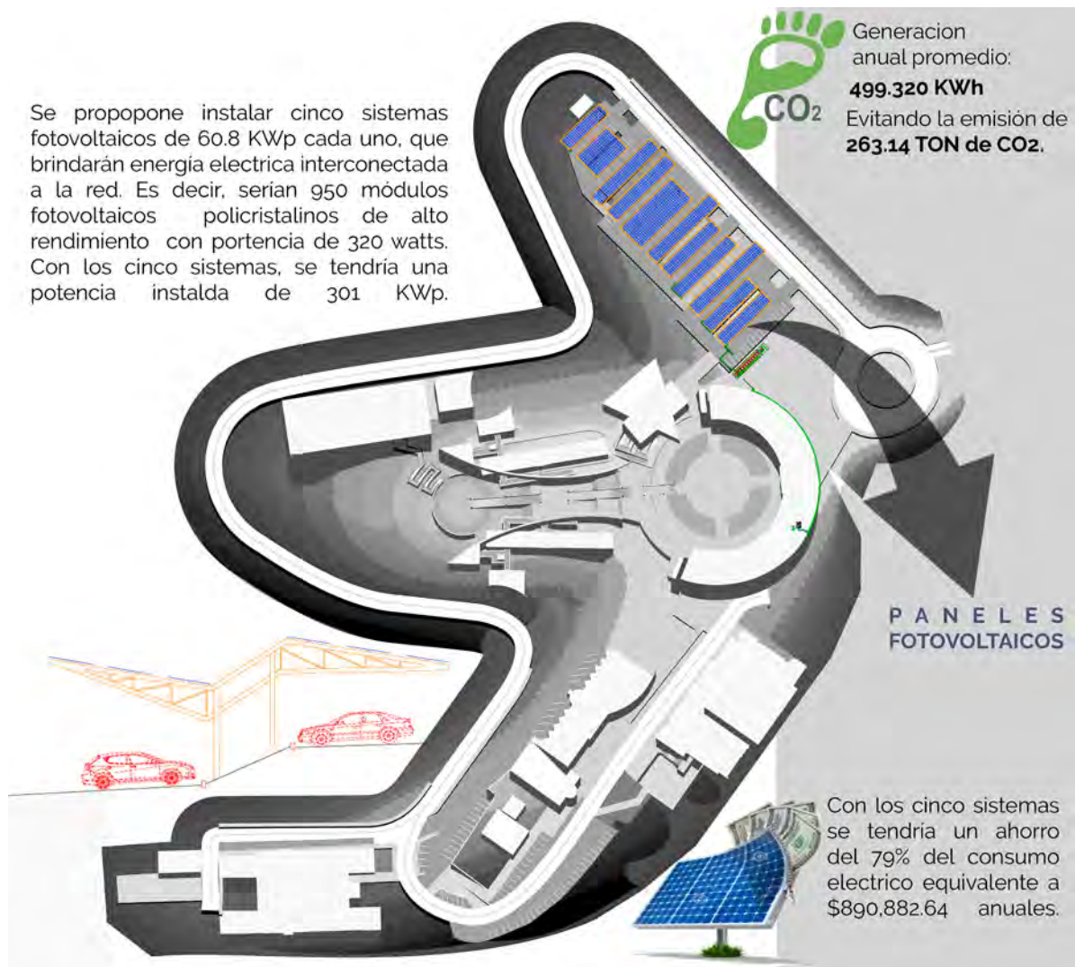
Imagen 5.8 Proyecto de Ahorro Energético en la Sede Marfil "Proyecto de implementación de un sistema de generación de energía eléctrica a través de energía solar fotovoltaica con interconexión a la red en la Sede Marfil"
