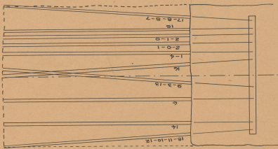
BARRENACION CON CURVA "V" PARA CRUCEROS DE 1.80x2.40 MTS. 3.40 AVANCE
