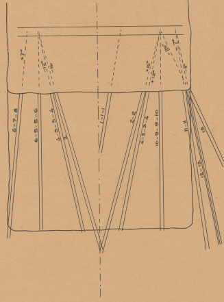
BARRENACION CON CURVA "V" PARA CRUCEROS DE 1.80x2.40 MTS. 1.60 AVANCE
