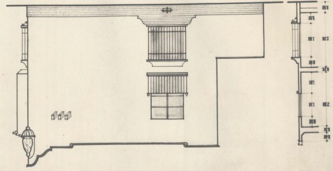
CASA TIPO-B1 FACHADA LATERAL.
