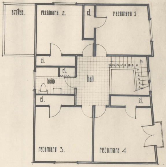
PLANTA ALTA. POSIBILIDAD DE 4 RECAMARAS.
