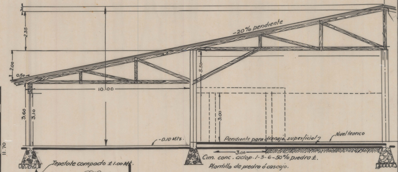
MEDIA SECCION TRANSVERSAL. -ESC.= 1:100.
